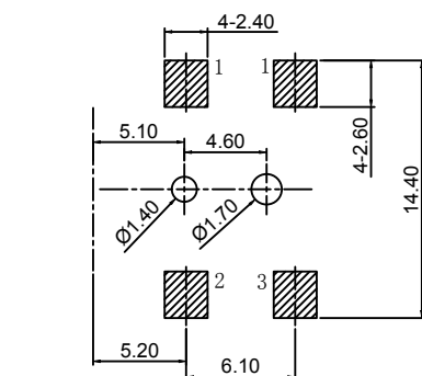
P.C.B 设计参考尺寸
